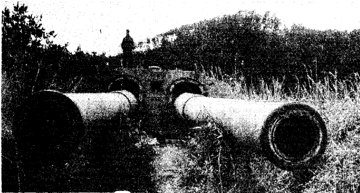
Fig. 13. 41-cm Turret
